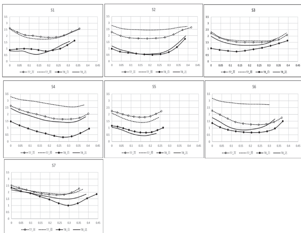
図3. 「百，搭，白，達」のピッチ曲線
