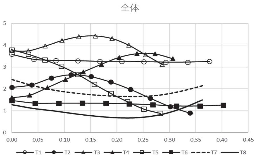
図2. 単字調のピッチ曲線（T値）
